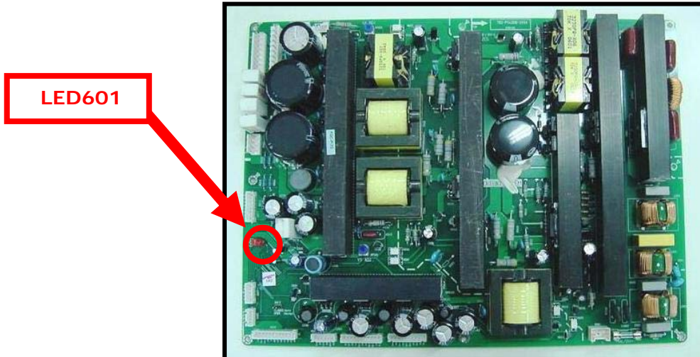
PCI FONTE PLASMA 3ª GERAÇÃO (95A3400001901)
