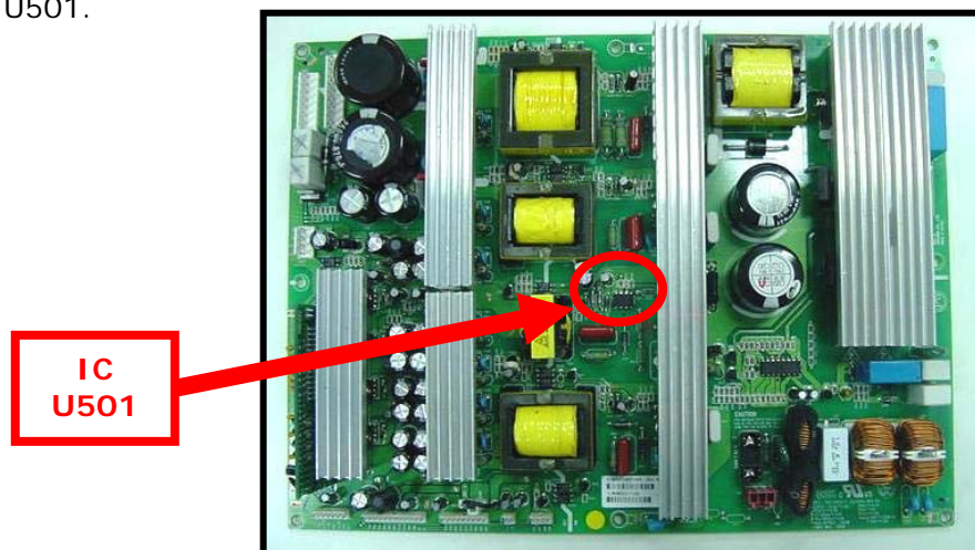
PCI FONTE PLASMA 1ª GERAÇÃO (95A0550001901)
