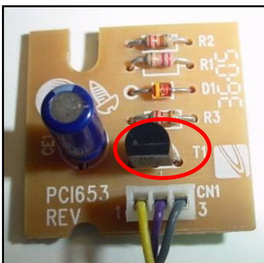
PCI RESET - Vista Superior (transistor T1 em destaque).
