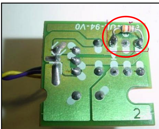
PCI RESET MODIFICADA - Vista Inferior (resistor de 3K9 soldado da base do T1 para o terra).
