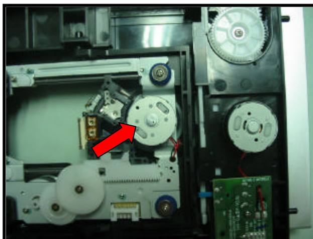
VISTA INFERIOR DO MECANISMO VERSÃO 1127. (MOTOR SPINDLE SEM ETIQUETA AZUL).
