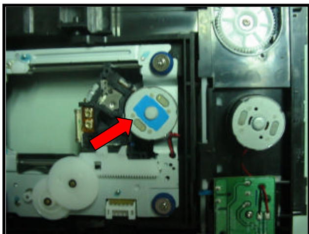
VISTA INFERIOR DO MECANISMO VERSÃO 1120. (MOTOR SPINDLE COM ETIQUETA AZUL).
