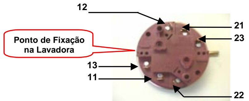
Figura 1: Pressostato Vermelho
