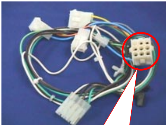
Conector de 9 vias 32.6001.21.4
