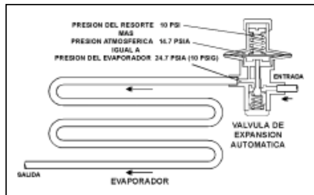
Figura 6.2 - Evaporador con válvula de expansión automática.
