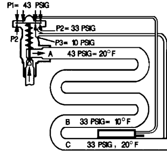
Válvula de Termo Expansión con igualador externo en un evaporador con una caída de presión de 10 psi.
