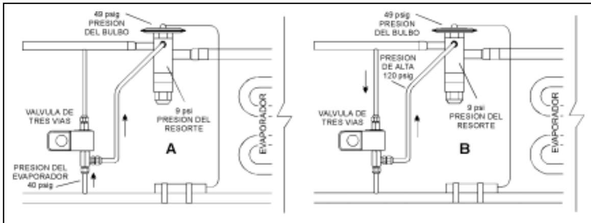
Figura 7.15 - Válvula de solenoide de tres vías utilizada para mantener la VTE herméticamente cerrada durante los ciclos de paro del compresor.
