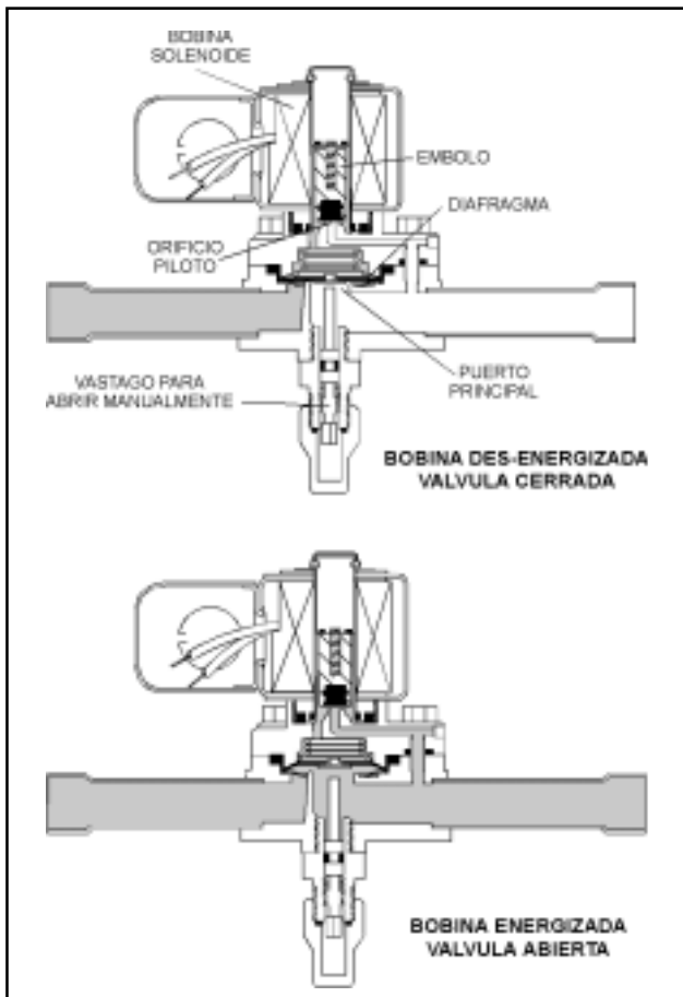
Figura 7.7 - Válvula de solenoide de dos vías operada por piloto, normalmente cerrada, con diafragma flotante.
