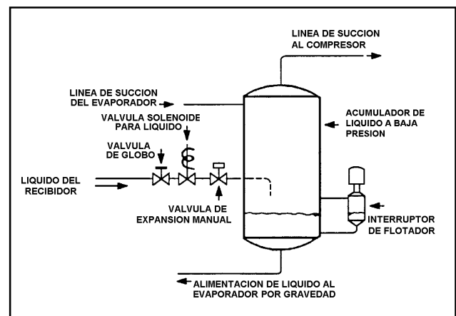
Figura 7.21 - Solenoide para alimentación de líquido.
