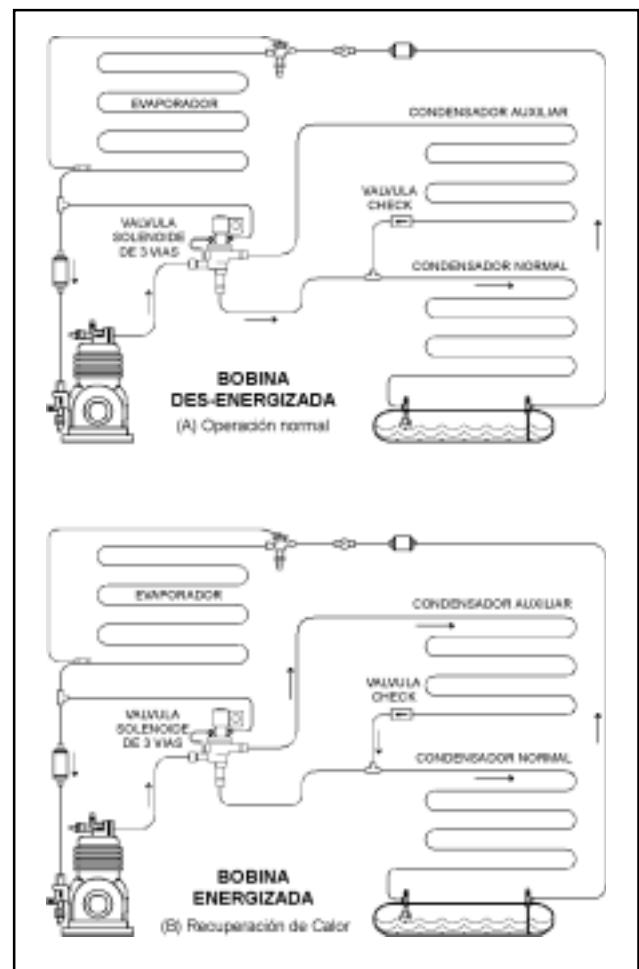
Figura 7.11 - Sistema de recuperación de calor, condensadores en serie.
