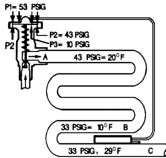
Válvula de Termo Expansión con igualador interno en un evaporador con una caída de presión de 10 psi.
