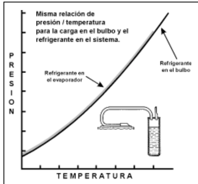
Figura 6.31 - Curvas de saturación típicas de una carga líquida.
