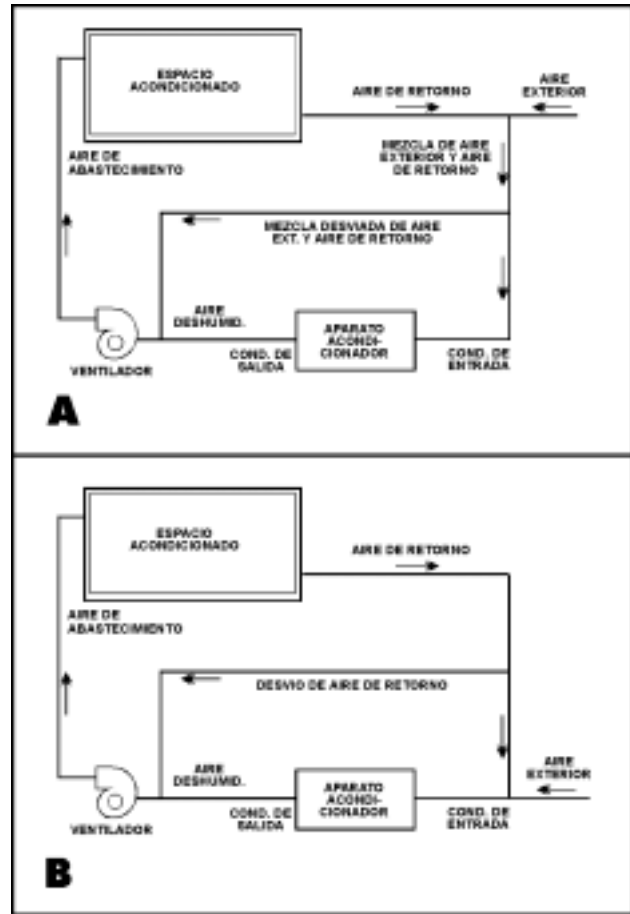
Figura 13.24 - Dibujos esquemáticos de los sistemas de desvío de aire. "A", desvío de una mezcla de aire exterior y aire de retorno; "B", desvío de aire de retorno solamente.
