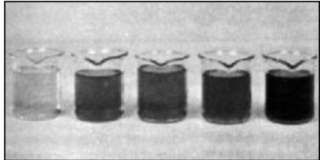
Figura 11.1 - Muestras de aceite tomadas de motocompresores con quemaduras leves.
