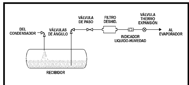
Figura 3.3- Ubicación más usual de un indicador de líquido y humedad.
