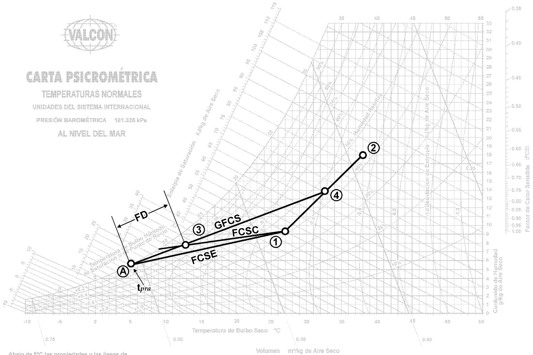
Figura 13.27 - Líneas de FCSC, GFCS y FCSE.
