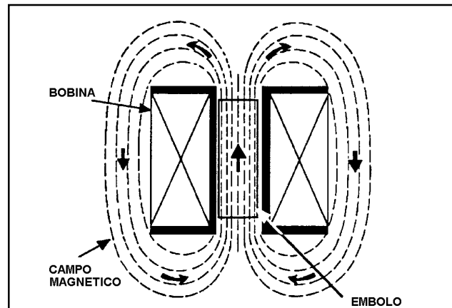
Figura 7.1 - Solenoide energizado.
