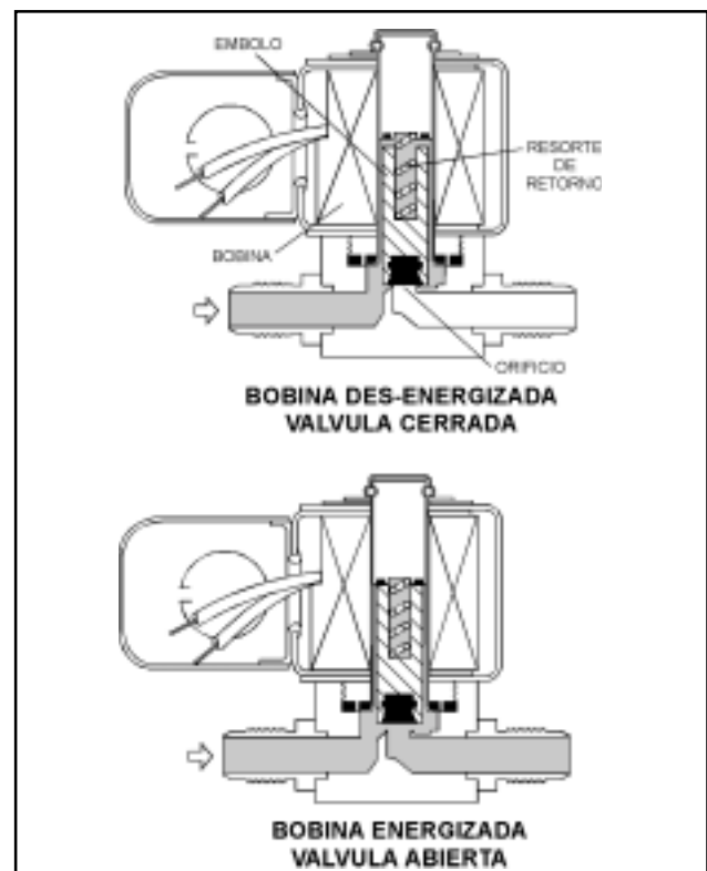
Figura 7.6 - Válvula de solenoide de dos vías, de acción directa, normalmente cerrada.
