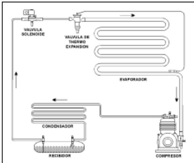
Figura 7.19 - Aplicación típica de una válvula de solenoide para línea de líquido.
