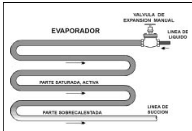
Figura 6.1 - Evaporador con válvula de expansión manual.
