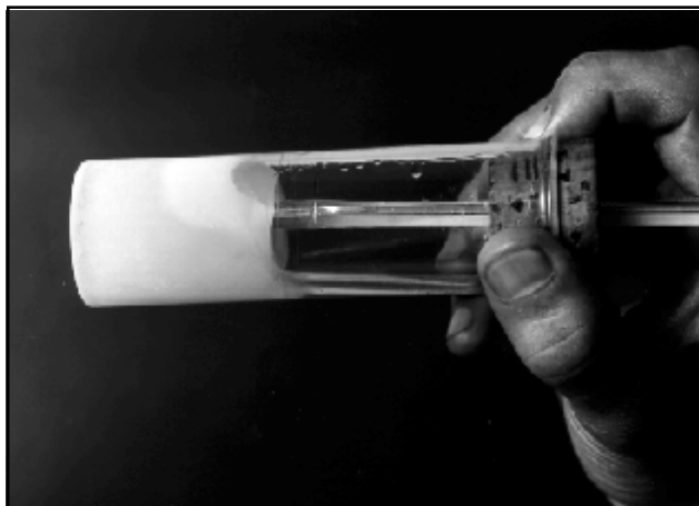
Figura 10.4- Aparato utilizado para determinar el punto de escurrimiento.
