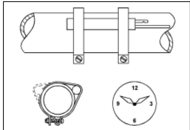
Figura 6.24 - Ubicación del bulbo remoto en líneas de succión de 7/8" a 1-5/8" de diámetro.
