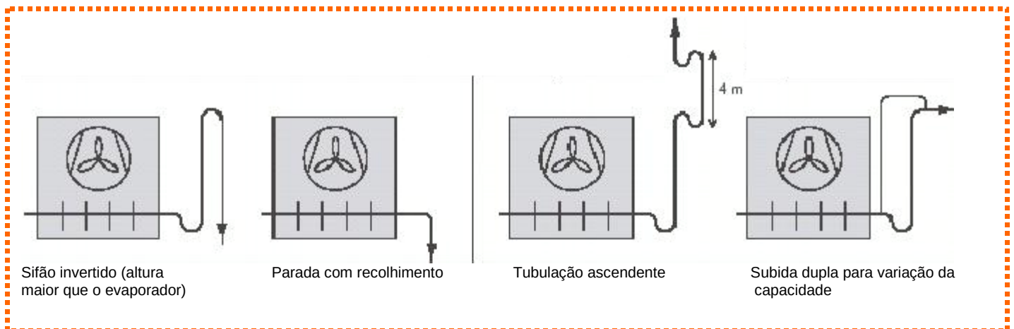
Figura 2: Lay out do tubo de sucção na saída do evaporador.
