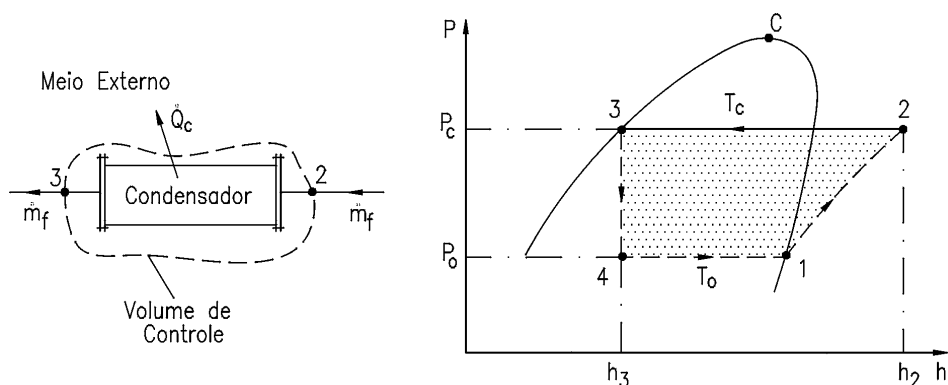
Figura 3.8 – Processo de transferência de calor no condensador.
