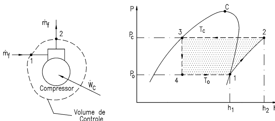
Figura 3.5 – Processo de compressão adiabático reversível no compressor.
