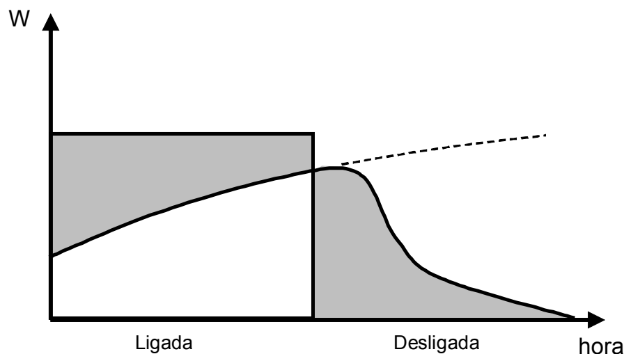
Figura 5.8: Relação entre carga térmica instantânea e real devido às lâmpadas.
