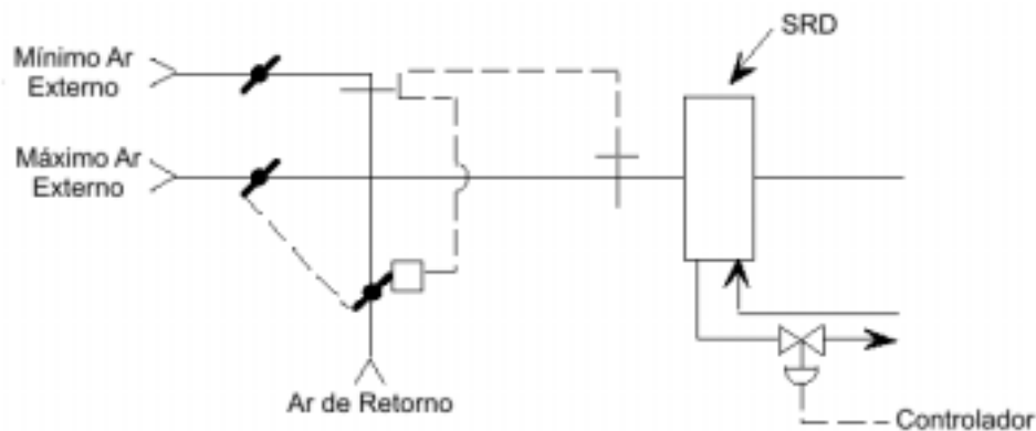
Figura 9.1 – Ciclo Economizador (por temperatura) – Controle da Temperatura de Mistura.
