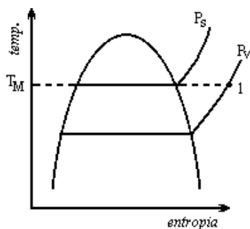
Figura 6.2 -Diagrama T x s para o ar.
