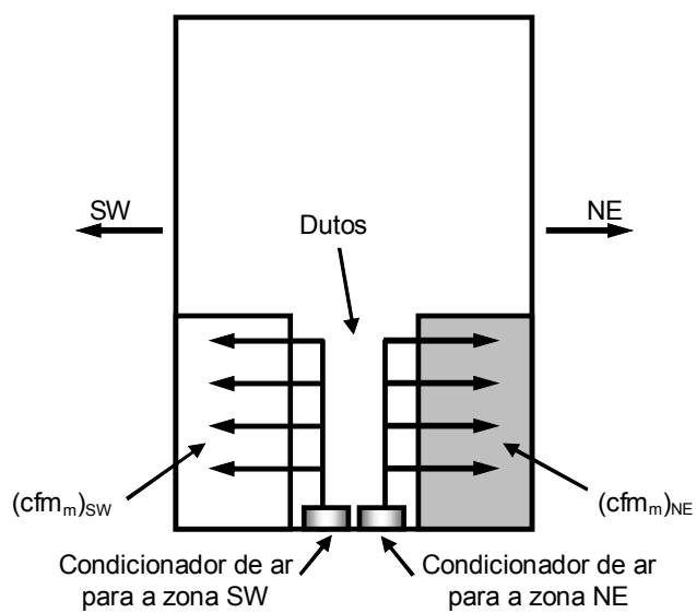
Figura 5.12: Ambientes atendidos individualmente.
