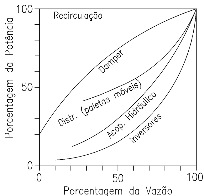
Figura 9.4 – Comparação entre diversos sistemas de controle de ventiladores centrífugos
