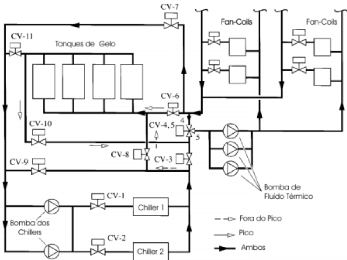
Figura 8.1 – Sistema de termocumulação com banco de gelo (internal-melt ice storage system).
