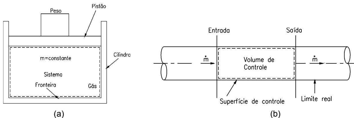
Figura 2.3 – (a) Sistema Fechado e (b) Sistema aberto (volume de controle).
