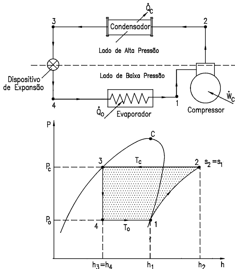
Figura 3.1 - Ciclo teórico de refrigeração por compressão de vapor.
