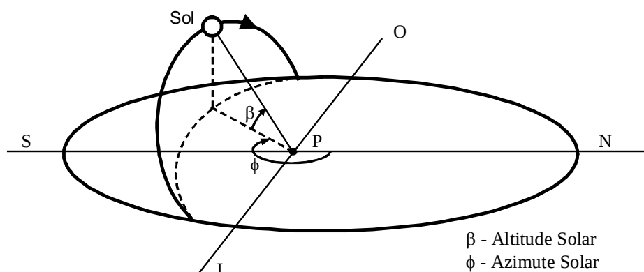
Figura 5.3: Ângulos de altitudes e azimuth solar.
