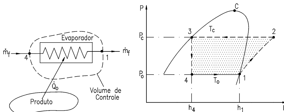
Figura 3.3 – Processo de transferência de calor no evaporador.
