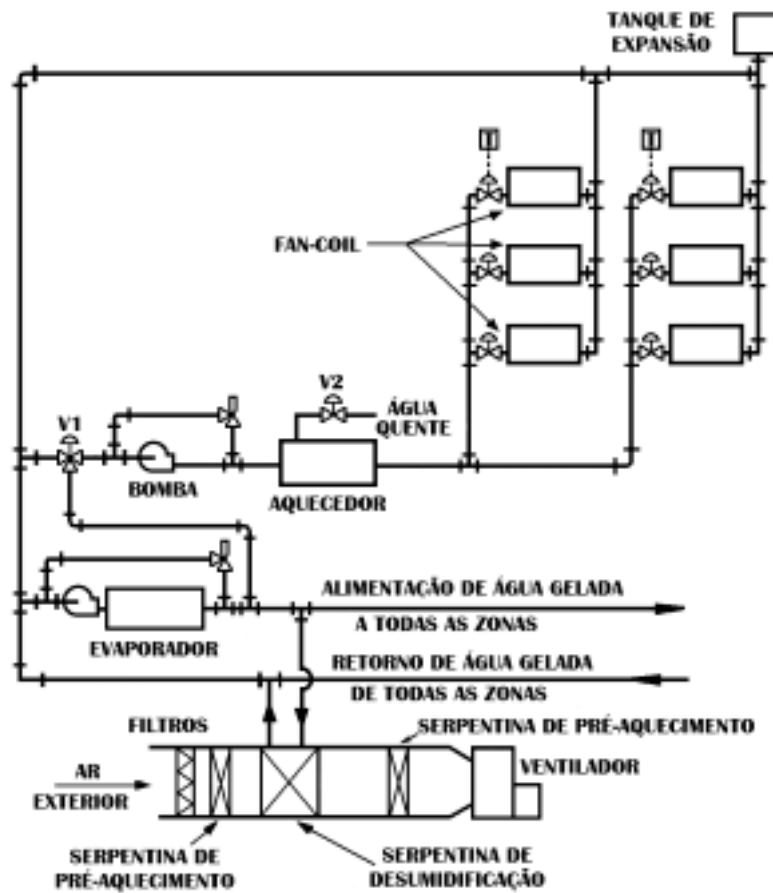
Figura 7.18, Instalação de fan-coil a dois tubos com ar primário.
