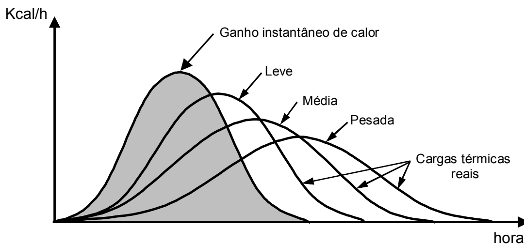
Figura 5.9: Efeito do peso da construção no armazenamento de calor.
