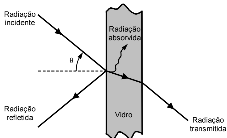
Figura 5.6: Radiação solar incidente sobre uma superfície de vidro.
