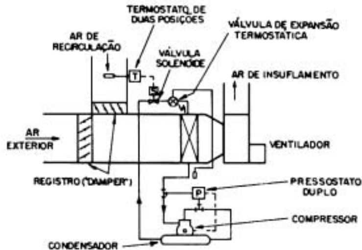
Figura 7.1. Instalação de Expansão Direta Com Regulagem Tudo-Nada.
