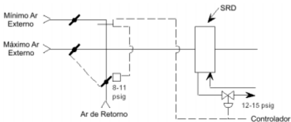
Figura 9.2 – Ciclo Economizador (por temperatura) – Controle da Temperatura da Água.
