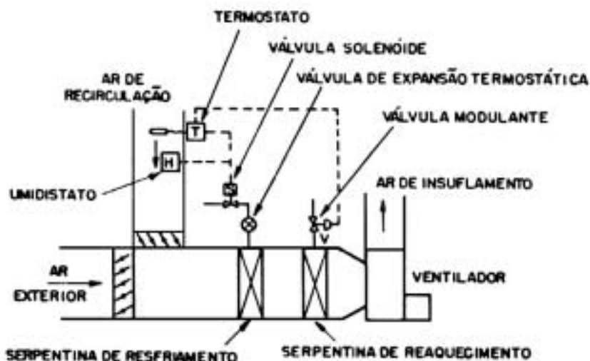
Figura 7.3. Instalação de Expansão Direta Com Reaquecimento.
