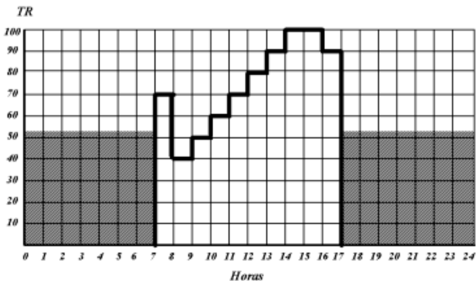
Figura 8.4: Sistema de armazenagem total.
