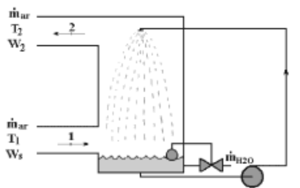
Figura 6.3 - Saturador Adiabático.
