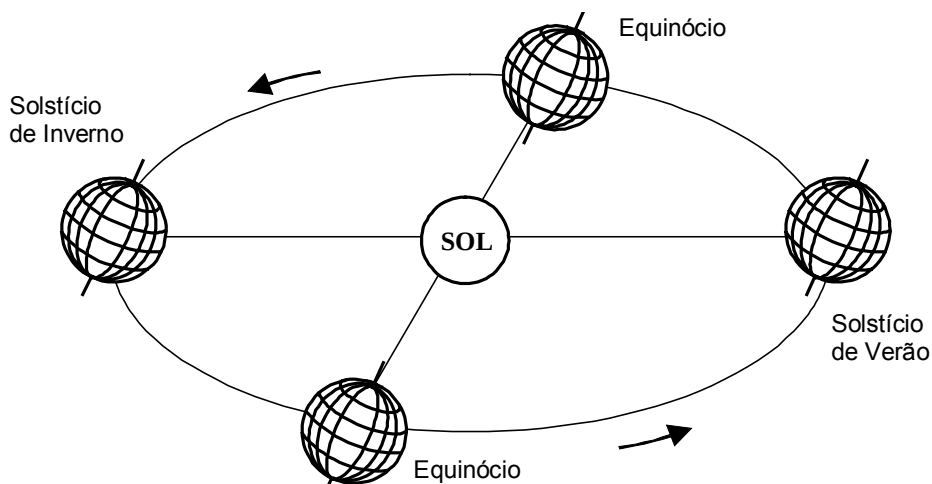
Figura 5.1: Movimento da terra em torno do sol.
