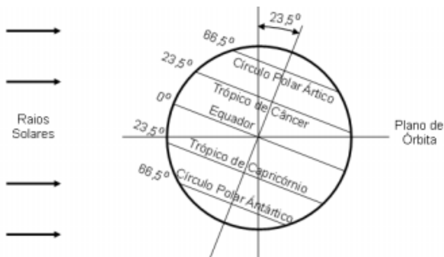
Figura 5.2: Solstício de verão hemisfério sul.
