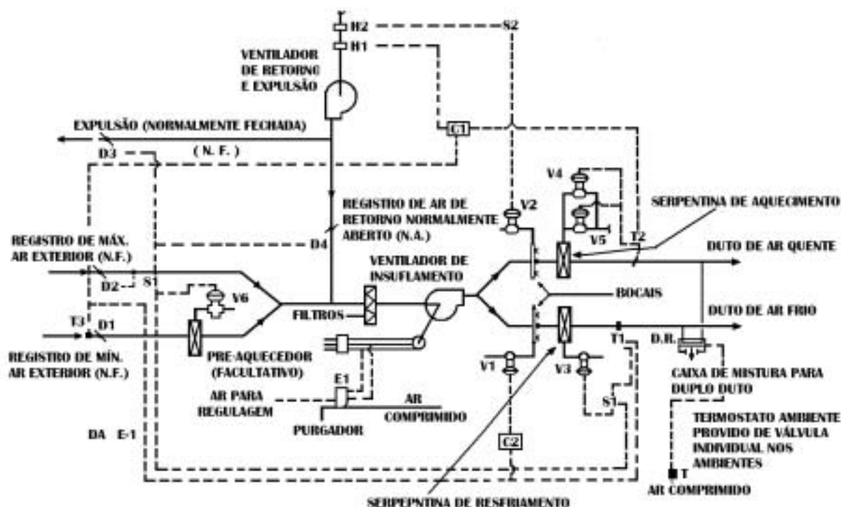
Figura 7.9. Esquema de controle para uma instalação de do tipo duplo duto.
