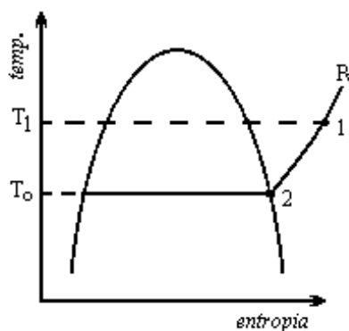
Figura 6.5 - Temperatura de orvalho ( T_o ).
