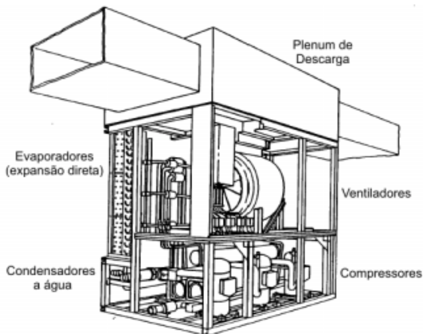
Figura 7.28. Self Contained (condicionador autônomo).
