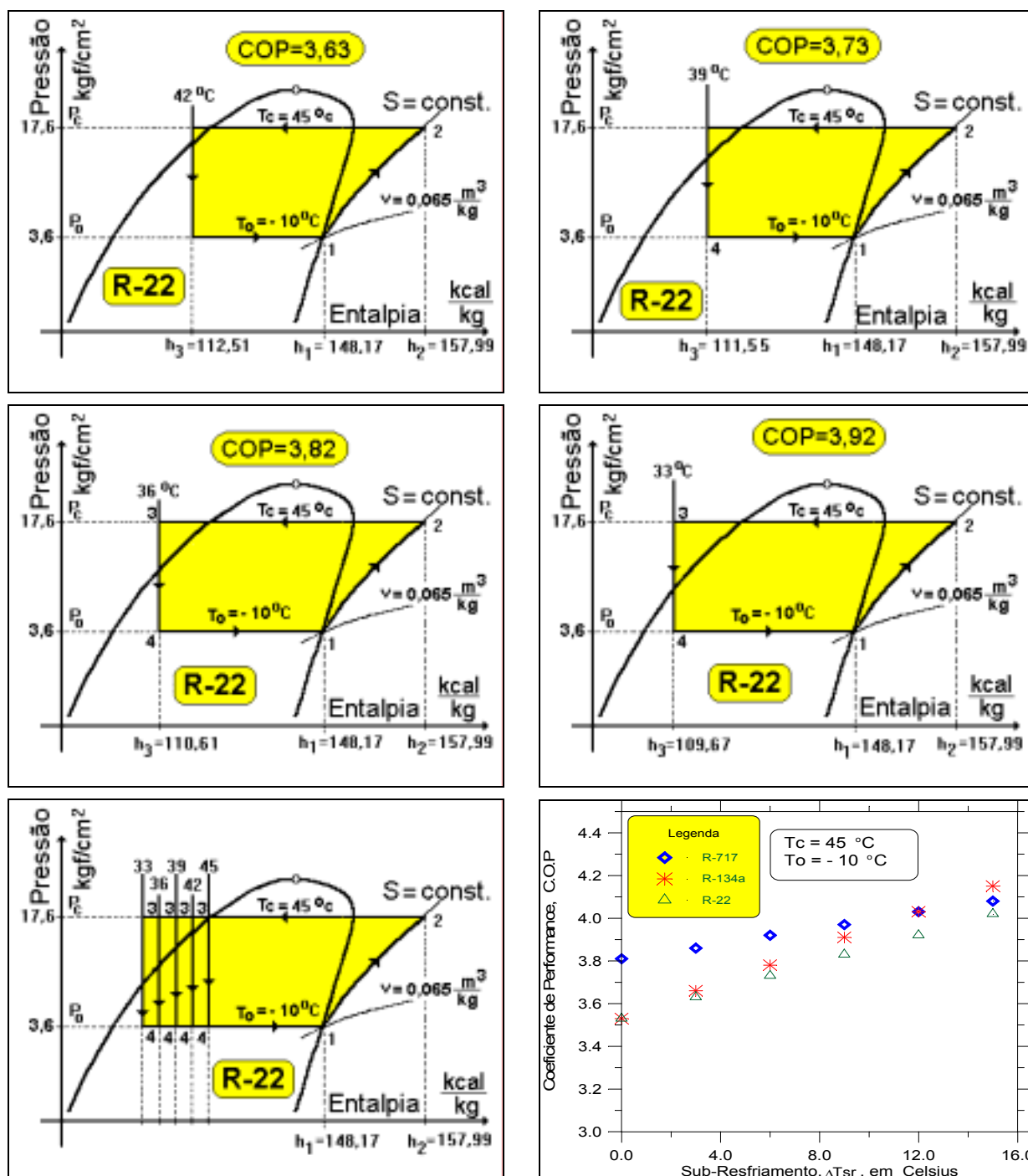
Figura 3.13 – Influência do sub-resfriamento no COP do ciclo teórico.
