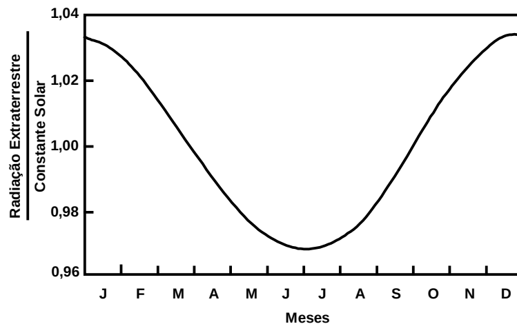
Figura 5.5: Relação entre a radiação extraterrestre e a constante solar.
