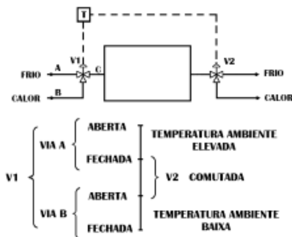
Figura 7.17. Instalação de indução a quatro tubos. Regulação dos indutores.
