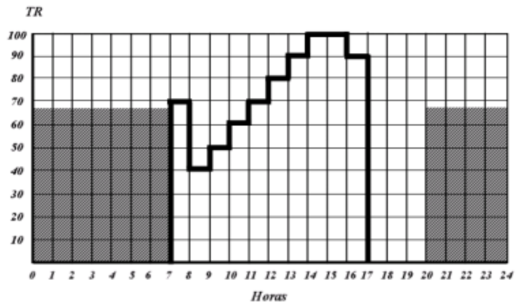
Figura 8.6 – Sistema de armazenagem parcial, com desligamento do chiller no horário de ponta.
