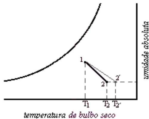
Figura 6.13- Desumidificação Química.
