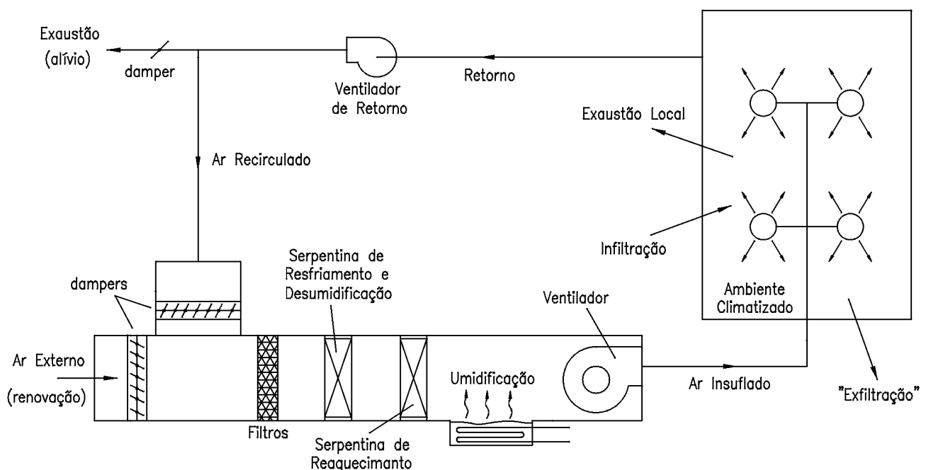
Figura 1.6 - Sistema de climatização típico.
