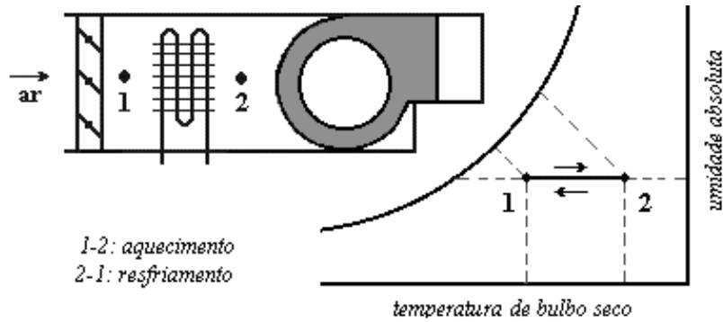
Figura 6.8 - Aquecimento e Resfriamento Sensível.
