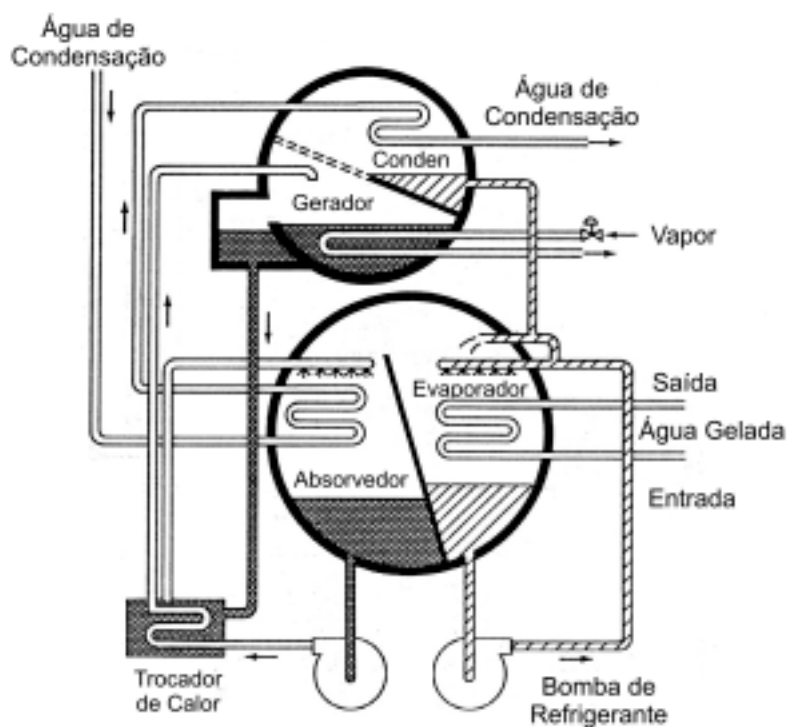
Figura 4.1 – Máquina de Refrigeração por absorção.
