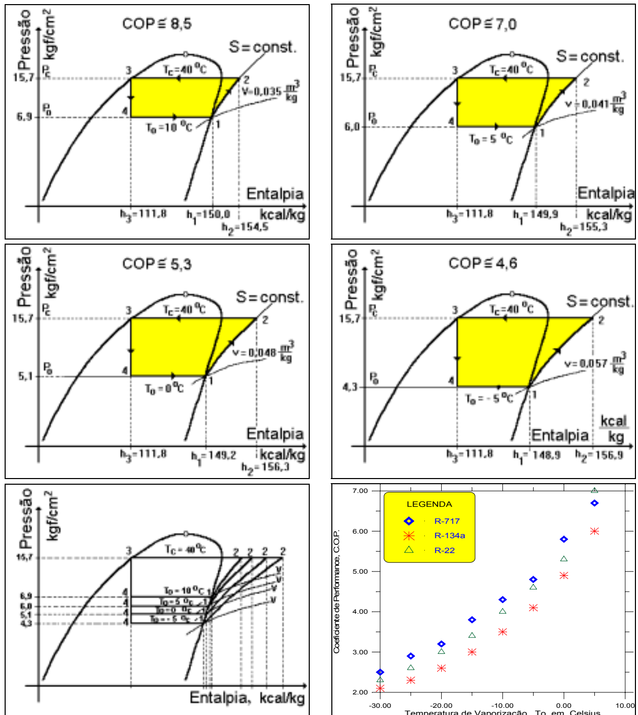
Figura 3.11 – Influência da temperatura de evaporação no COP do ciclo teórico.
