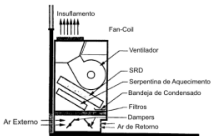
Figura 7.21 – Climatizador de ar do tipo Fan-Coil.
