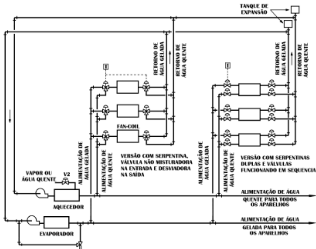
Figura 7.25. Instalação de fan-coils a quatro tubos.
