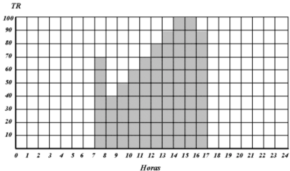
Figura 8.3: Perfil típico da carga de ar condicionado de um edifício comercial.
