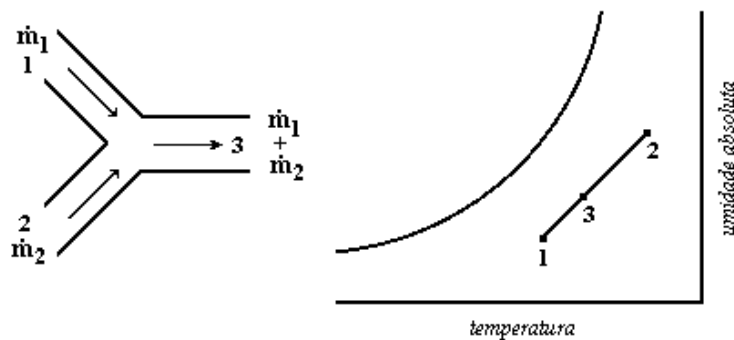
Figura 6.7 - Mistura adiabática de suas correntes de ar.
