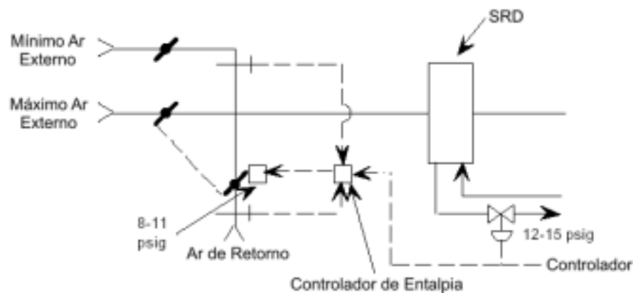
Figura 9.3. Ciclo Economizador (por entalpia) – Controle da Temperatura da Água gelada.
