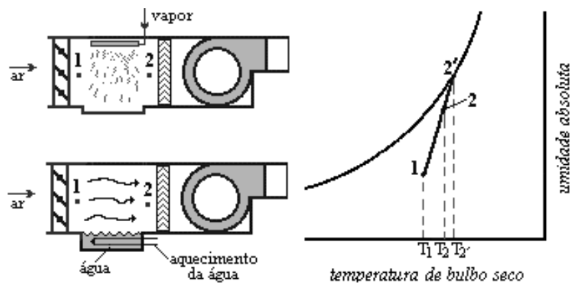
Figura 6.12 - Aquecimento e Umidificação.
