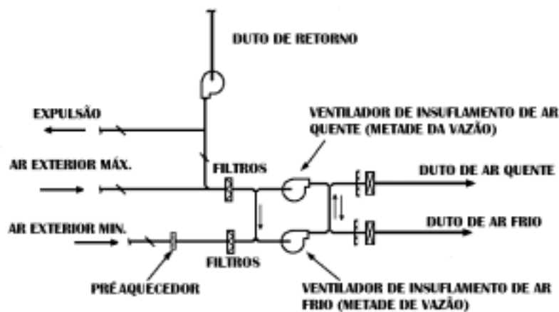
Figura 7.11. Instalação com dois ventiladores e uma serpentina de desumidificação na descarga de um deles.
