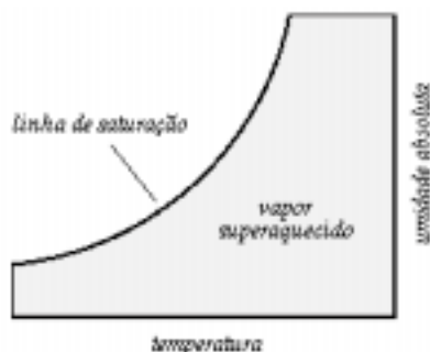
Figura 6.1 - Esquema de uma carta psicrométrica para o ar saturado.
