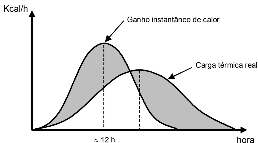
Figura 5.7: Defasagem entre a radiação solar instantânea e carga térmica real
