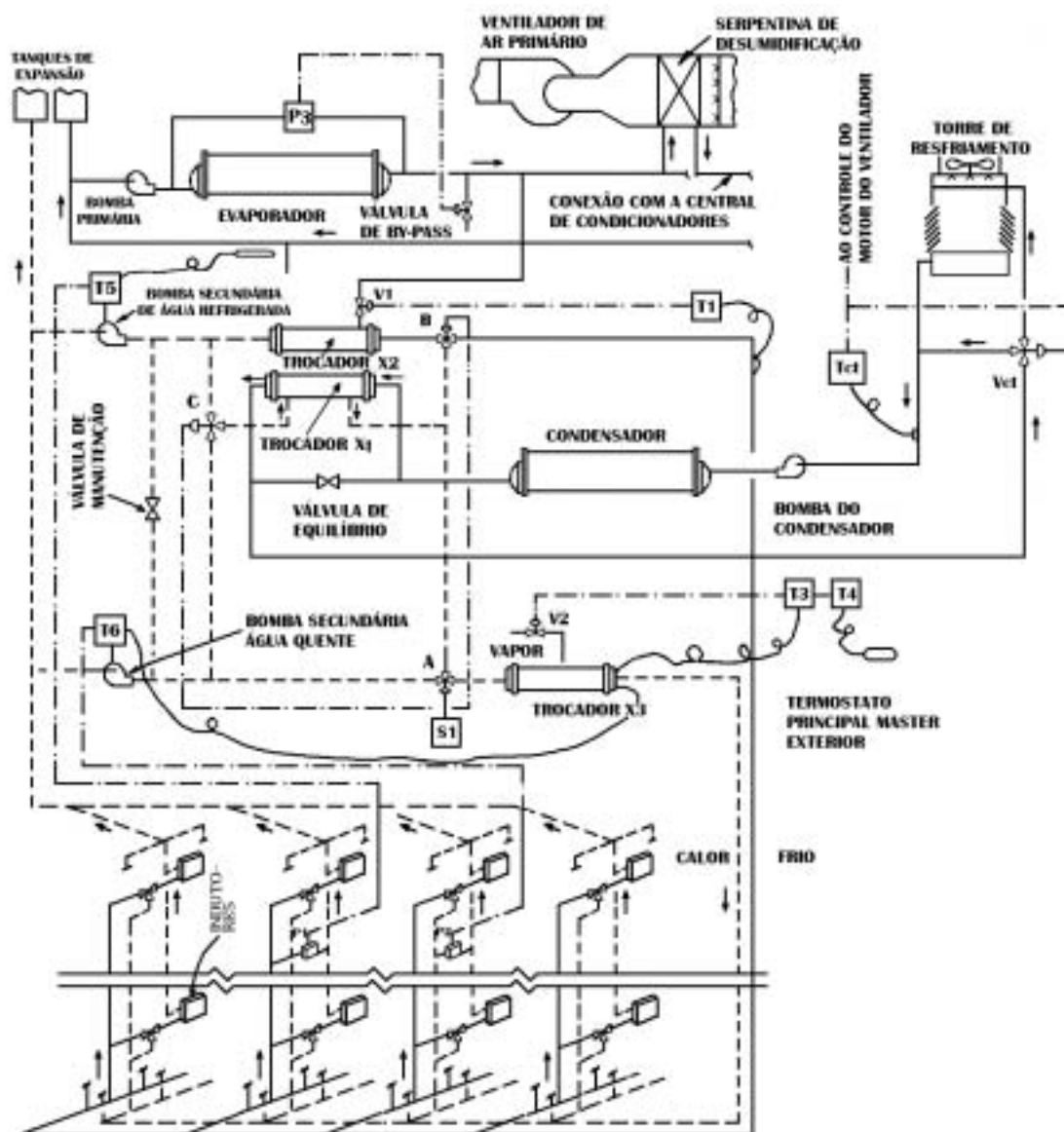
Figura 7.16. Instalação de indução a três tubos.
