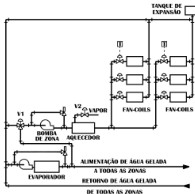
Figura 7.23. Instalação de fan-coils a dois tubos. Controle da temperatura pela variação da vazão de água.
