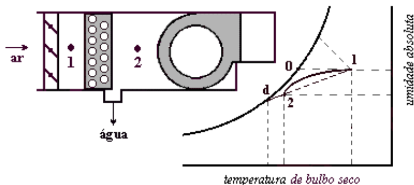
Figura 6.9 - Resfriamento e Desumidificação.
