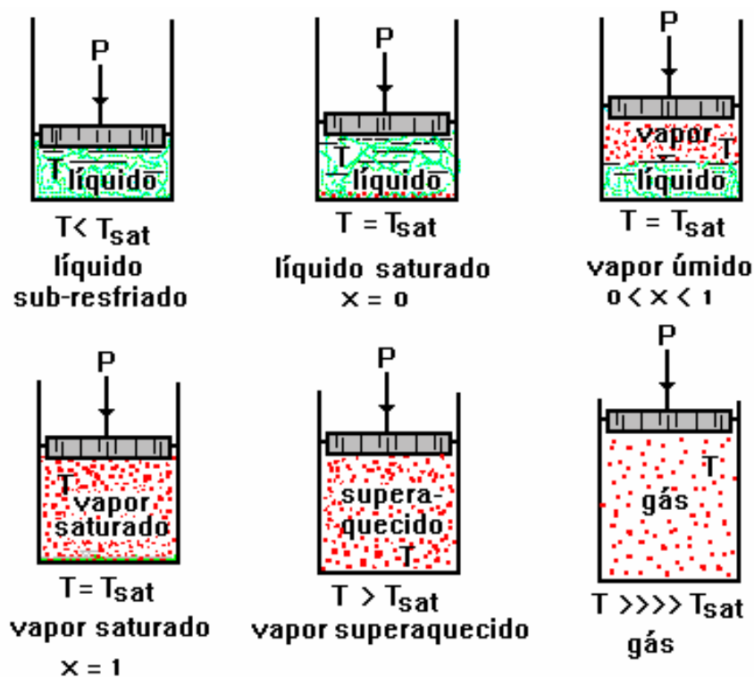
Figura 2.1 - Estados de uma substância pura.
