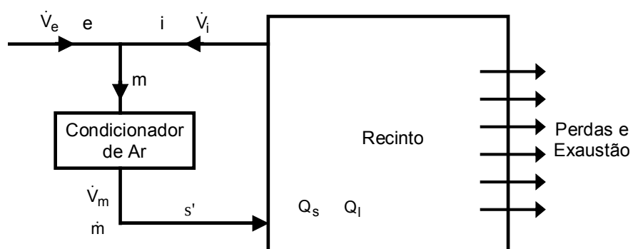
Figura 6.16 Sistema de ar condicionado padrão
