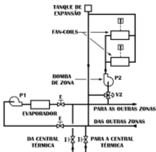
Figura 7.22. Instalação de fan-coils a dois tubos. Controle da temperatura pelo acionamento dos ventiladores.
