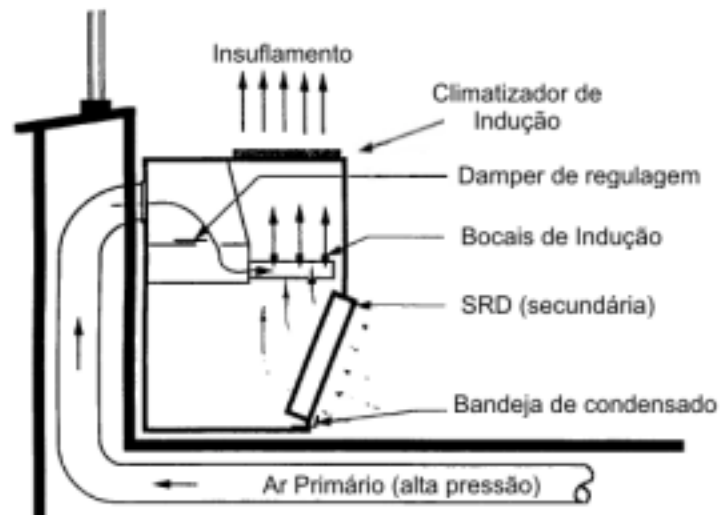
Figura 7.13 – Climatizador de Indução
