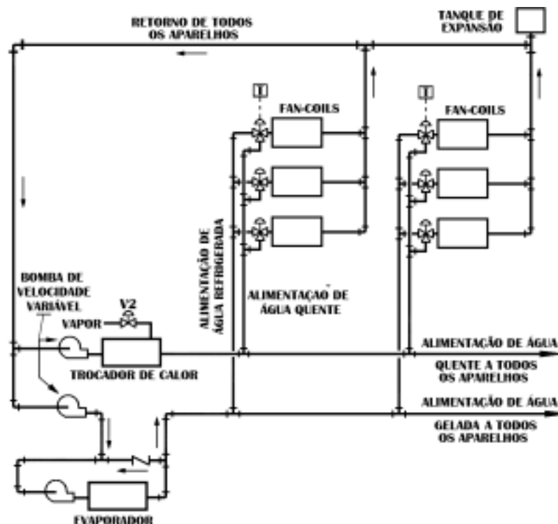
Figura 7.24. Instalação de fan-coil a três tubos.
