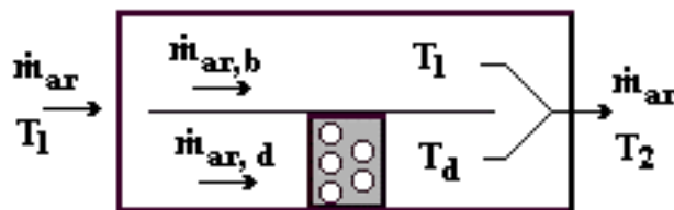
Figura 6.10 - Representação esquemática do Bypass de ar.
