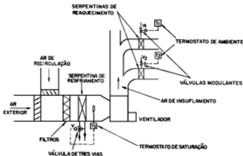
Figura 7.4. Instalação Com Reaquecimento Para Múltiplas Zonas.
