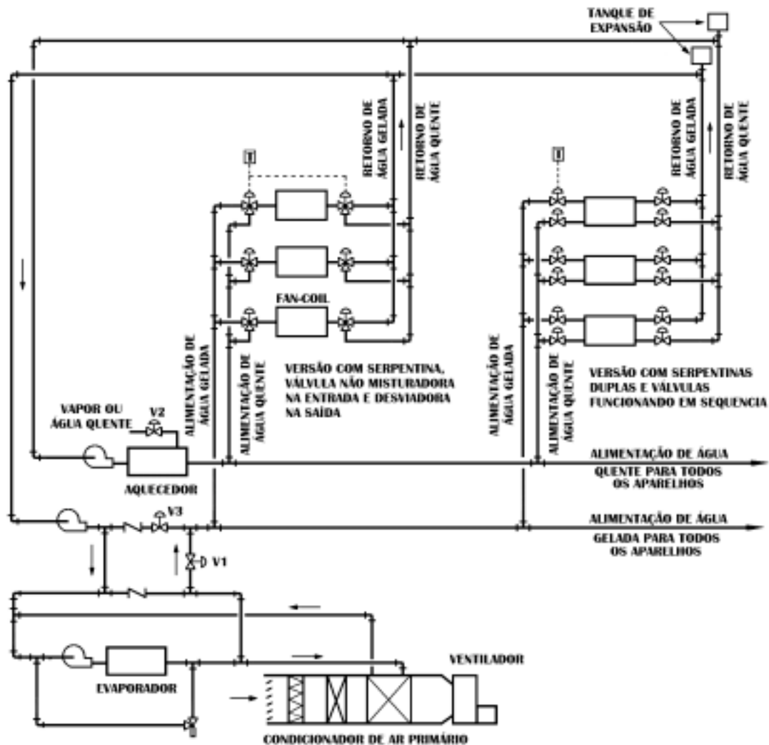
Figura 7.20. Instalação de fan-coils a quatro tubos com ar primário.
