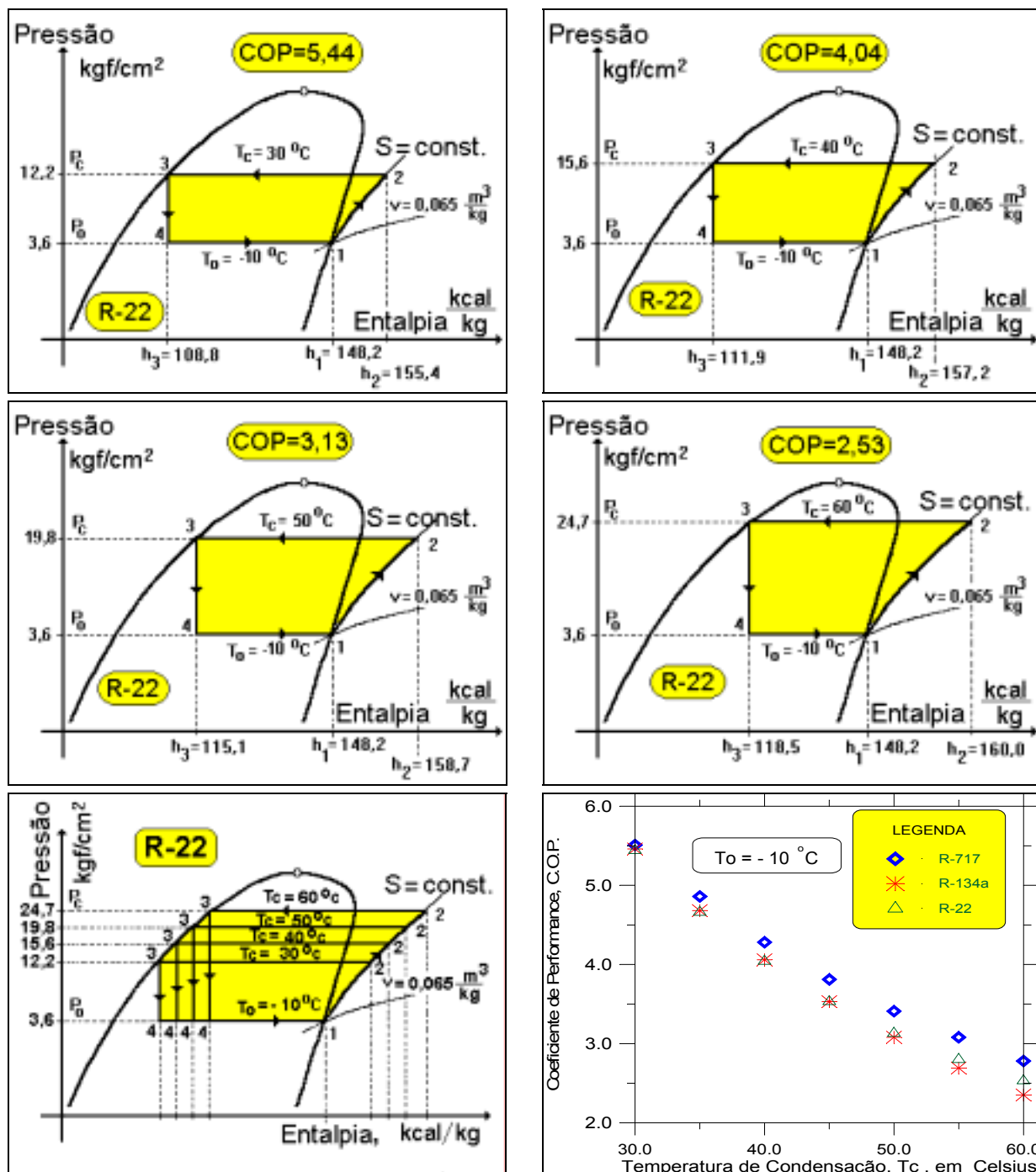
Figura 3.12 - Influência da temperatura de evaporação no COP do ciclo teórico.
