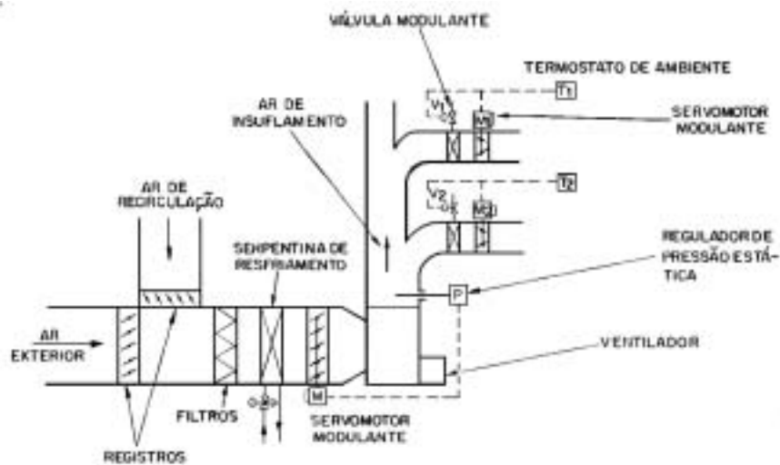
Figura 7.6. Instalação Com Variação de Vazão e Temperatura.
