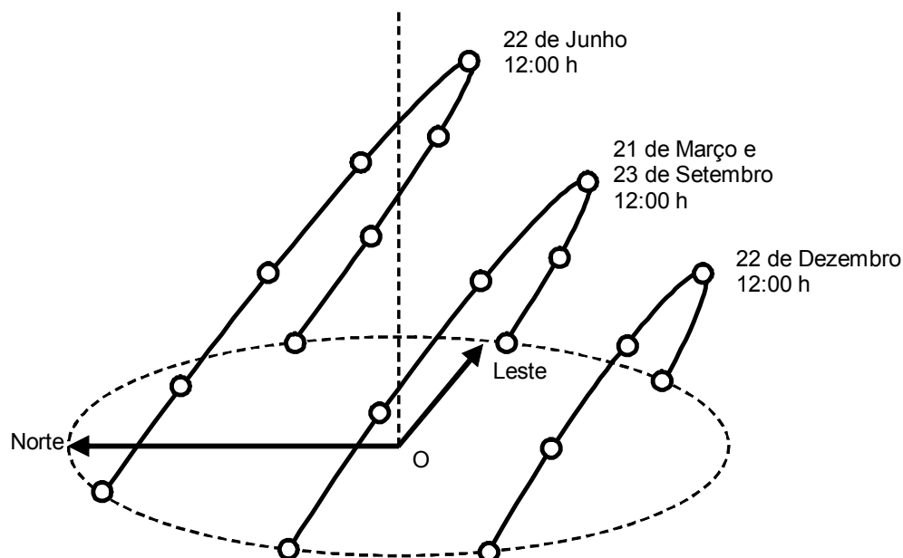
Figura 5.4: Caminhos aparentes do sol.
