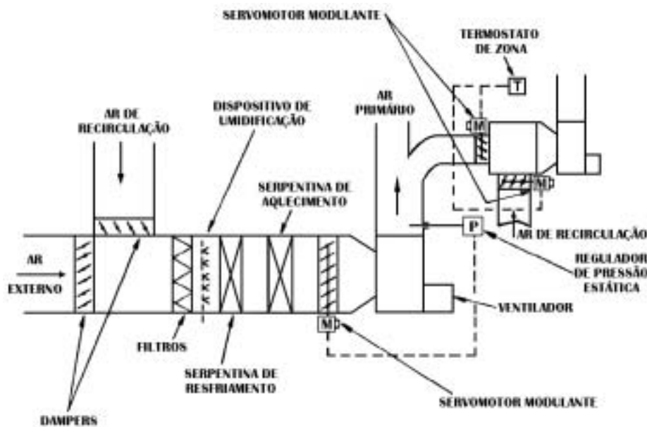
Figura 7.7. Instalação Com Vazão Variável e Recirculação Local
