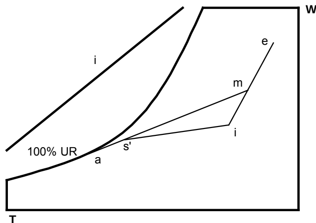
Figura 6.17: Evolução na carta psicrométrica - Sistema de ar condicionado padrão
