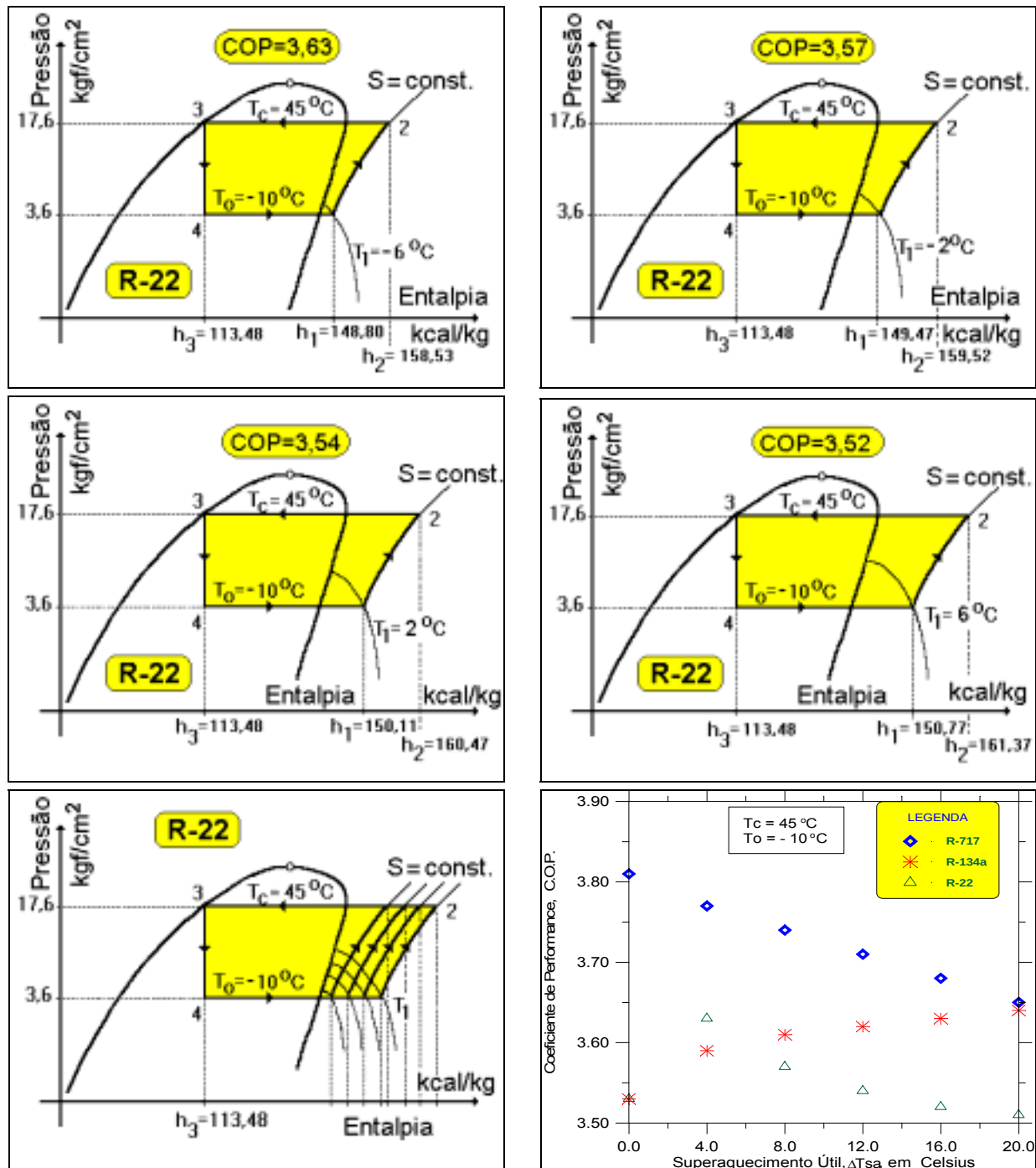
Figura 3.14 - Influência do superaquecimento no COP do ciclo teórico.
