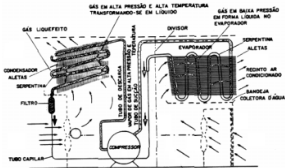
Figura 7.26 – Condicionador de ar de janela.
