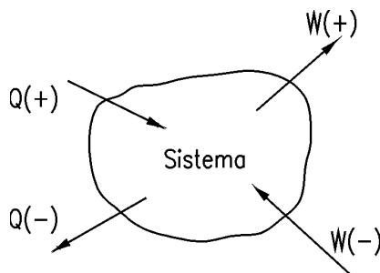
Figura 2.4 - Convenção dos sinais para trabalho e calor.
