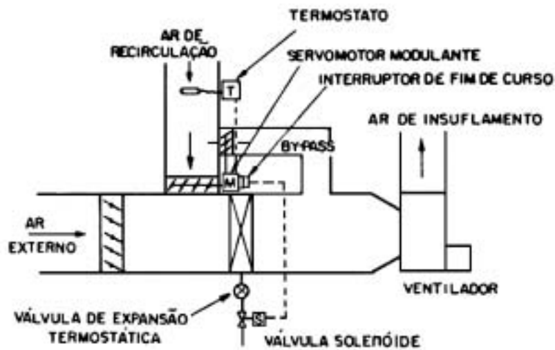
Figura 7.2. Instalação de Expansão Direta Com Bypass do Ar de Recirculação.
