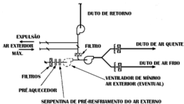
Figura 7.10. Instalação com somente um ventilador de insuflamento e serpentina de desumidificação na descarga do mesmo e na tomada de ar externo.
