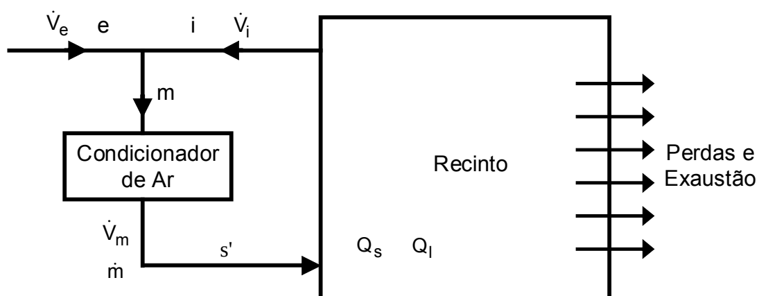
Figura 6.14: Desenho esquemático da instalação de ar condicionado.
