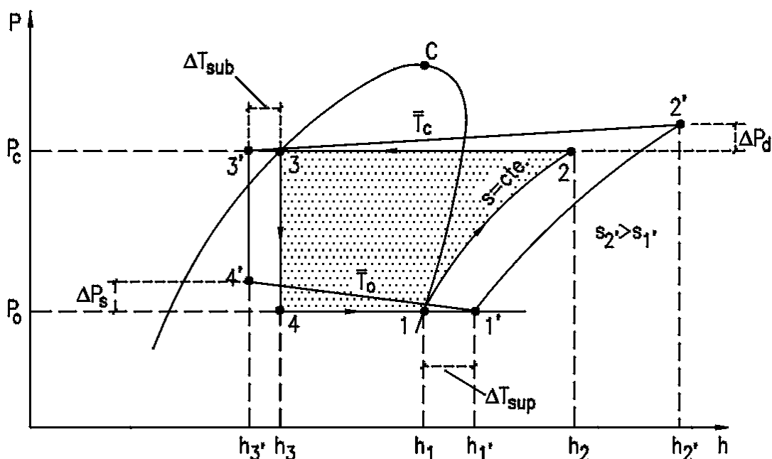
Figura 3.2 – Diferenças entre o ciclo teórico e o real de refrigeração.
